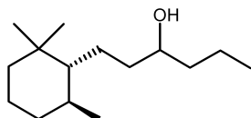
(+)-(3R)-1-[(1R,6S)-2,2,6-trimethylcyclohexyl]-3-hexanol
